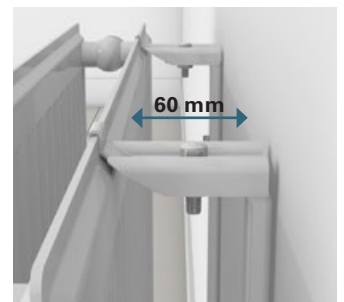
Wandabstand 60 mm genügend Platz für Reinigungs- und Desinfektionsmaßnahmen hinter dem Heizkörper
